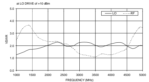
MCA-50LH VSWR
